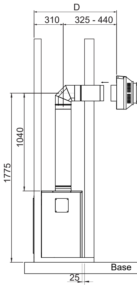
RDV3611 Long Horiz. Flue Kit B (R3661)
