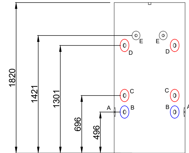
500L (MSX0500)
