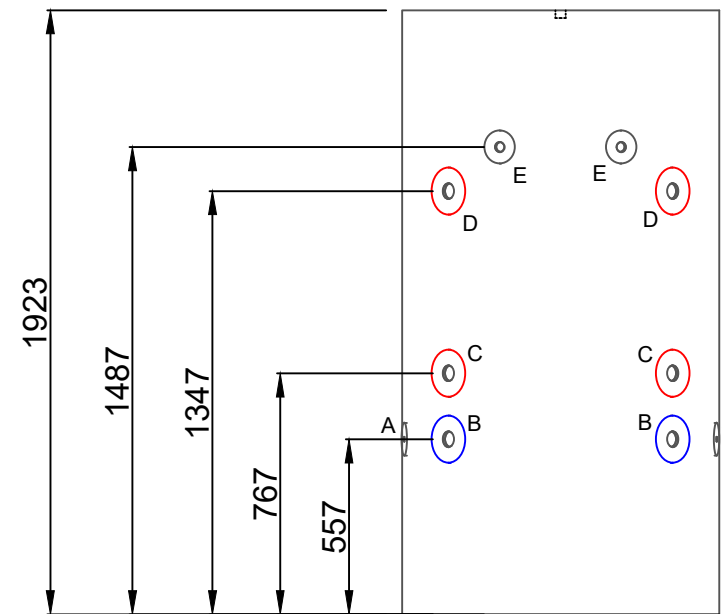
800L (MSX0800)
